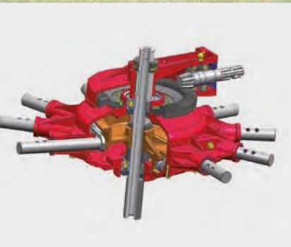
Olajfürdős hajtómű. (CompactLine)
